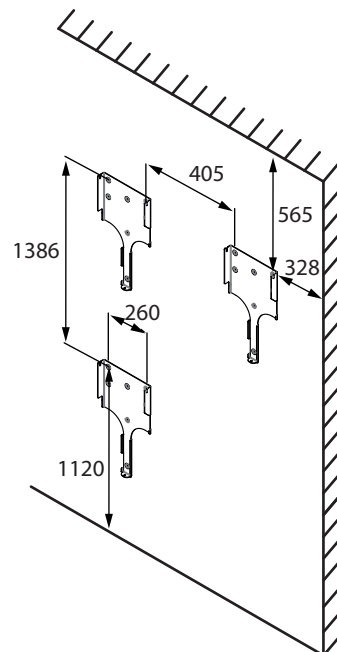
Σχήμα 3: Αποστάσεις διάτρησης (σε mm)
