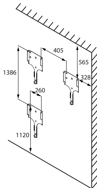
Figura 3: distanze di foratura (in mm)
