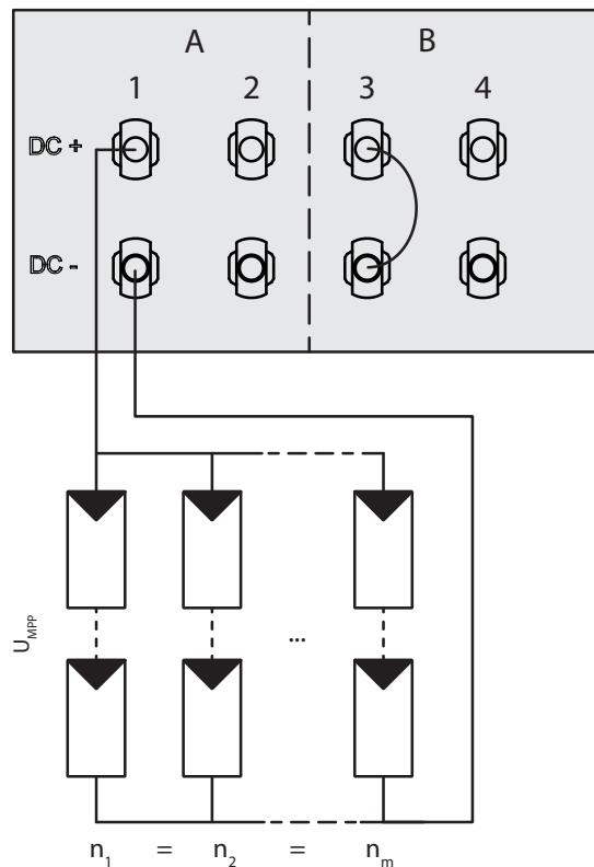
Afbbeelding 9: Parallele ingangsschakeling met Y-adapter, kortsluiting van de niet gebruikte MPP-tracker B
