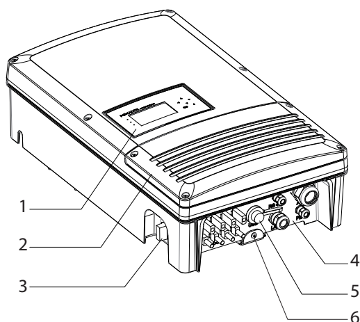
Obr. 1: Konstrukce střídače
