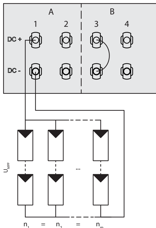
Figure 10 : Montage des entrées en parallèle avec adaptateur Y, court-circuitage du régulateur MPP B non utilisé
