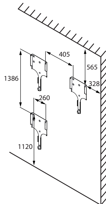
Afbeelding 3: Boorafstanden (in mm)
