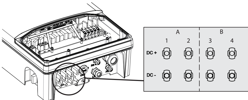
Slika 7: Priklučki za DC plus in DC minus
