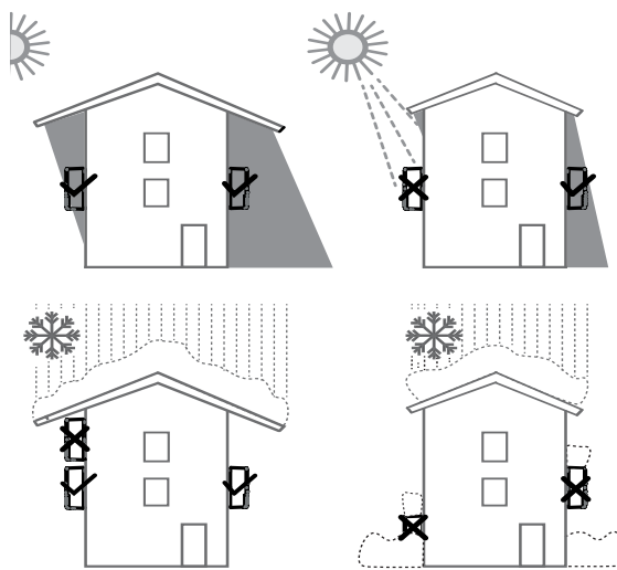
фиг. 4: Инвертор при инсталиране на открито
