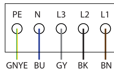
Afbeelding 6: AC-aansluitklemmen
