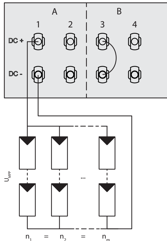
Billede 9: Parallel indgangskabling med Y-adapter, kortslutning af den ikke anvendte MPP-sporingsenhed B
