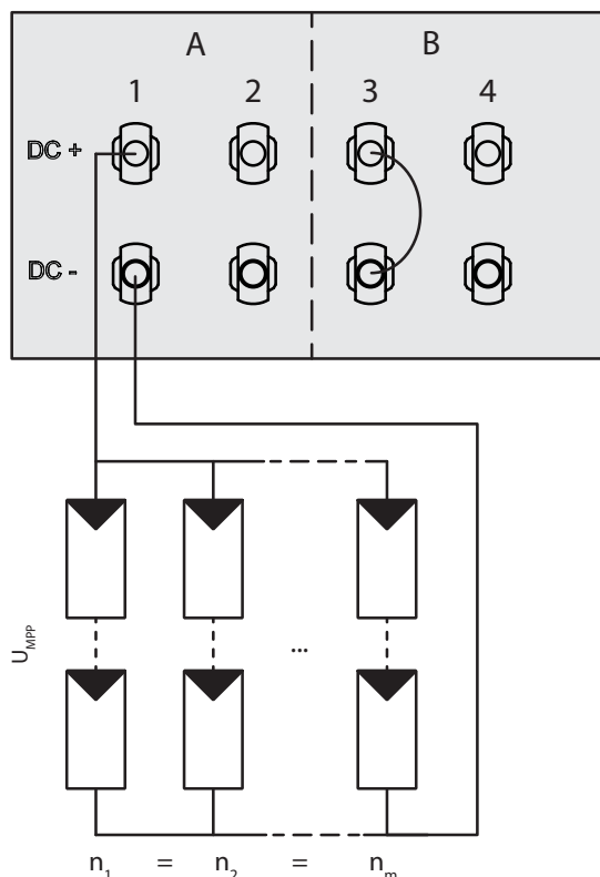
Figura 9: Ligação em paralelo com adaptador Y, curto-circuito no tracker MPP B não usado
