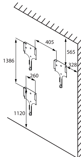
Billede 3: Boreafstande (i mm)
