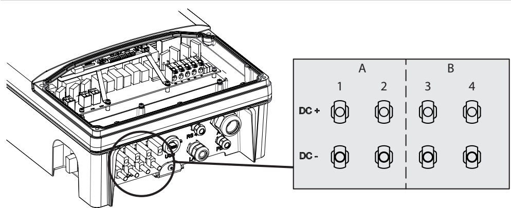
Figura 7: Conexiones para CC-positivo y CC-negativo
