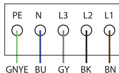
Σχήμα 6: Ακροδέκτες σύνδεσης AC
