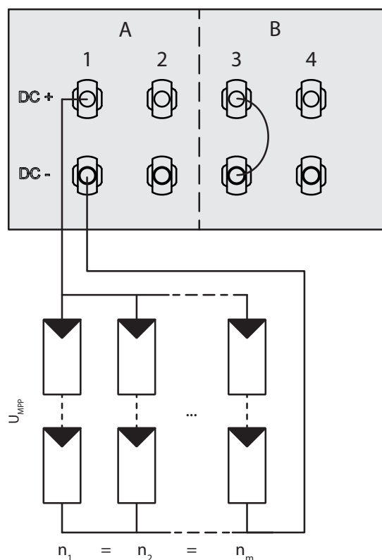
Slika 9: Vzporedna vezava vhodov z Y adapterjem, kratek stik MPP-sledilnika B, ki ni uporabljen
