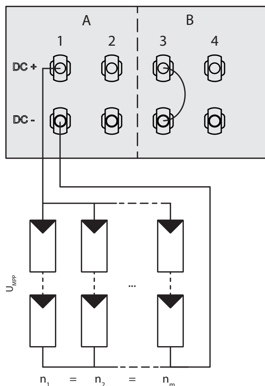
9. kép: Párhuzamos bemeneti kapcsolás Y-adapterrel, a nem használt MPP-követő B rövidzárata
