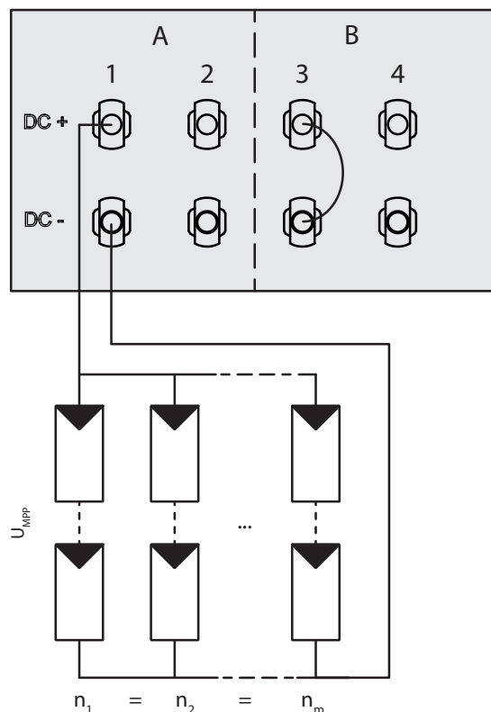
фиг. 11: Un générateur sur le 1er régulateur, 2e régulateur désactivé
