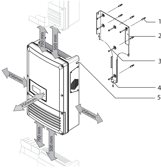
Şekil 5: Minimum mesafeler/montaj plakası
