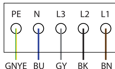
6. kép: AC csatlakozókapcsok
