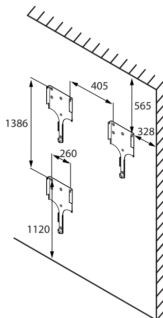
3. kép: Furatok távolsága (mm)
