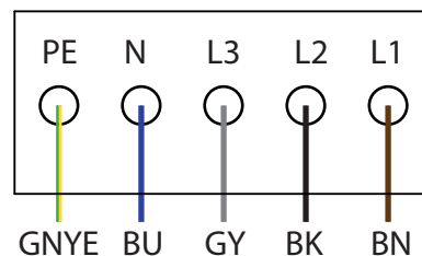
Rys. 6: Zaciski przyłączeniowe AC
