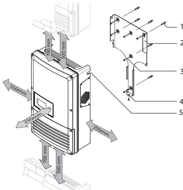
фиг. 5: Минимални разстояния/монтажна планка
