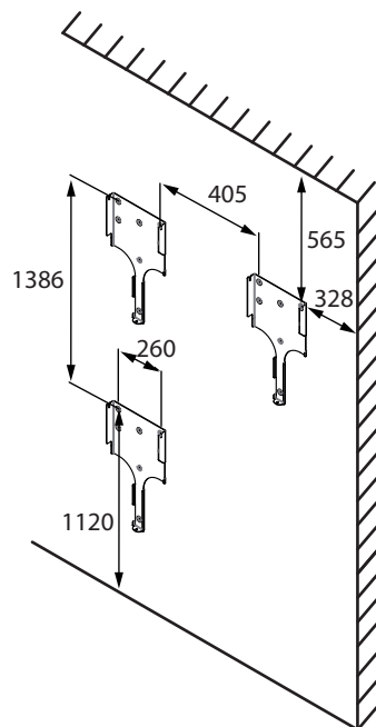
Slika 3: Razdalje med izvrtinami (v mm)
