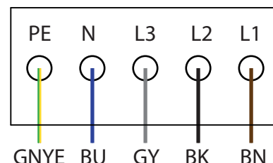
фиг. 8: АС присъединителни клемите
