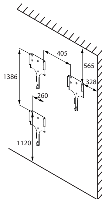
Figura 3: Distancia de agujeros (en mm)
