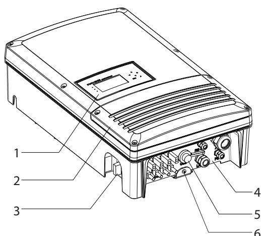
Figura 1: Estrutura do inversor
