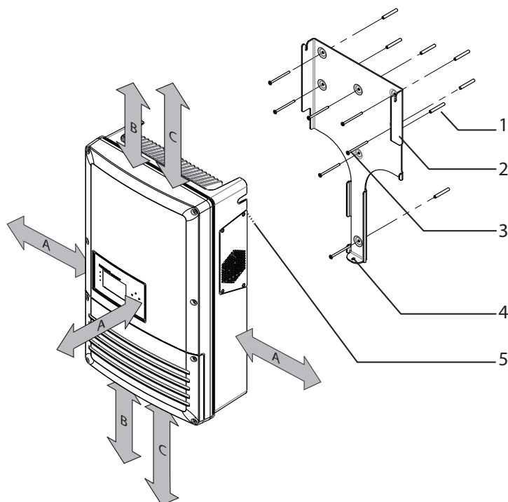
Figura 4: distanze minime / piastra di montaggio
