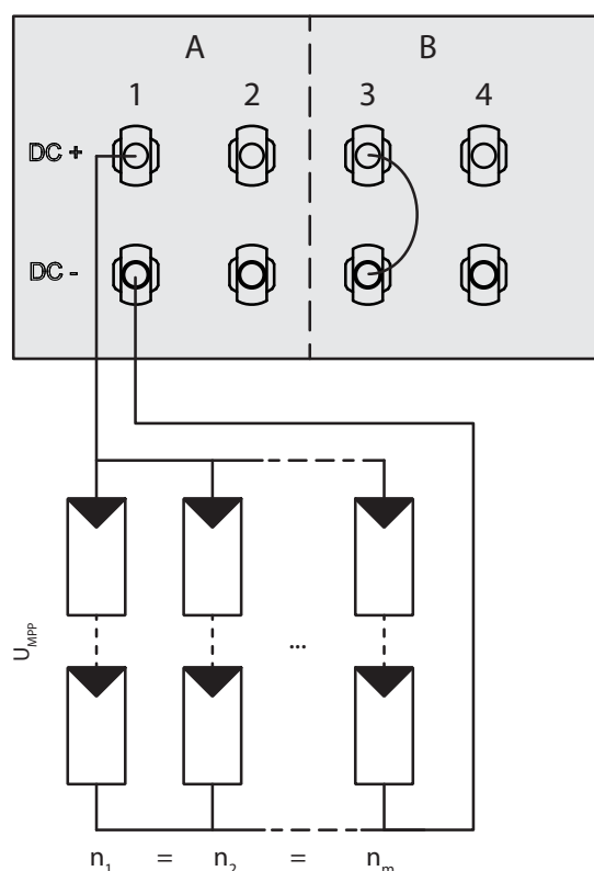
Rys. 9: Układ równoległy wejść z adapterem Y, zwarcie nieużywanego trackera MPP B
